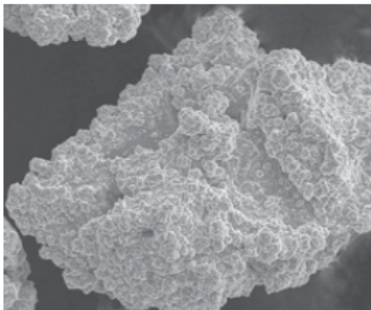
N56, N30(Cluster Type) Niコート: 30~60wt%
