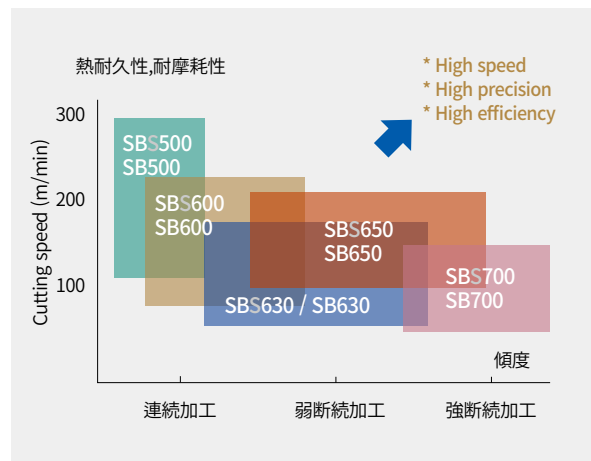
低cBN含有量PCBN切削条件
