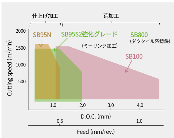
高cBN含有量PCBN切削条件
